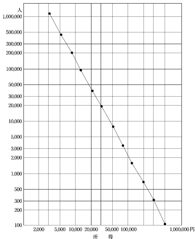
図4 パレート法則 (1945年, 日本)
