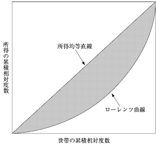
図1 ローレンツ曲線
