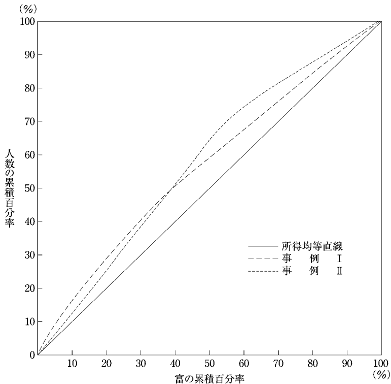
図7 ローレンツ曲線の交差
